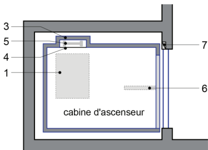
Grundriss
