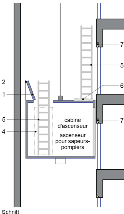
Schnitt
